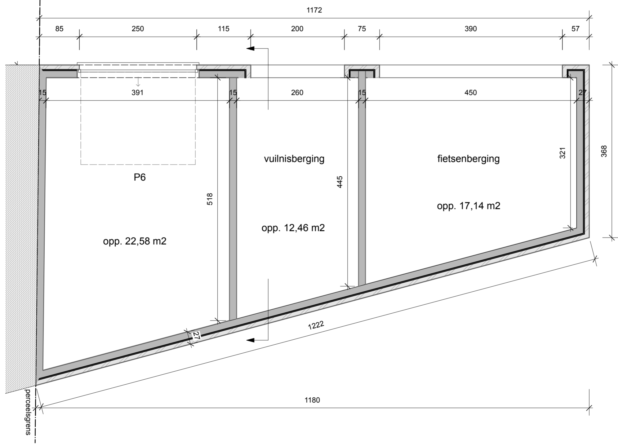
grondplan
